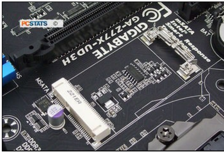
Conexión mSATA
