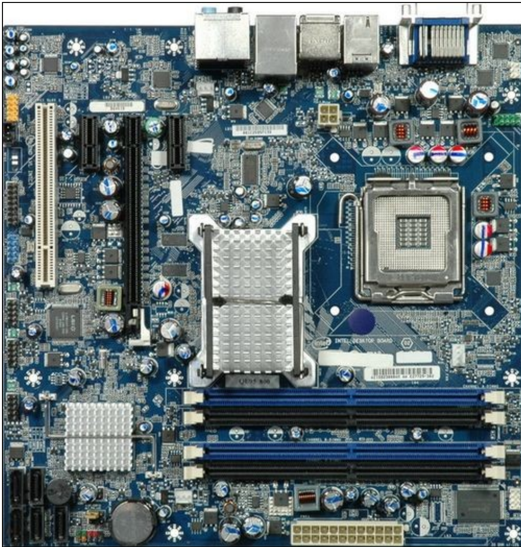
Placa INTEL microATX DG45ID do ano 2.008 para Micros com Socket-775.
