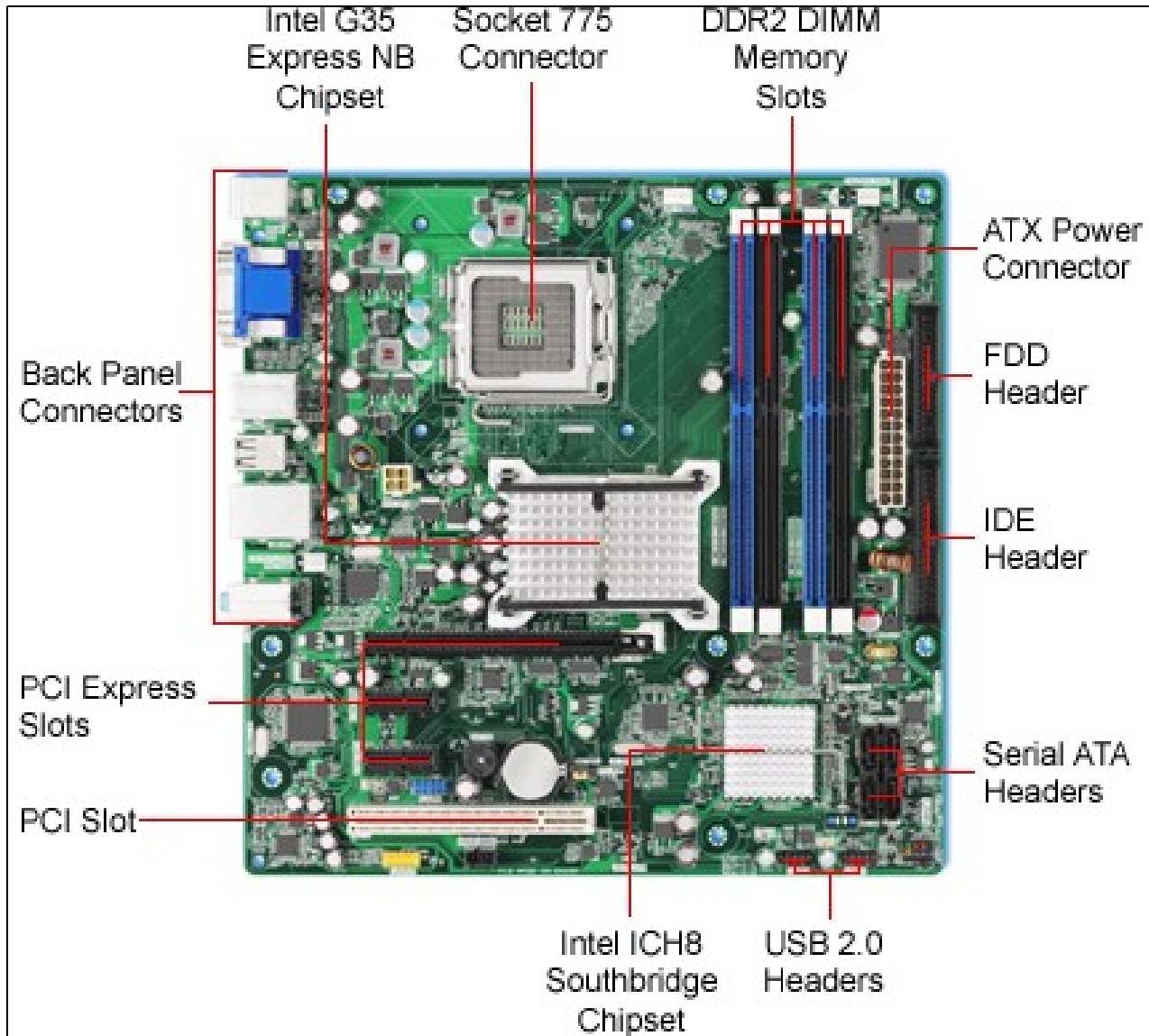
INTEL microATX DG35EC
